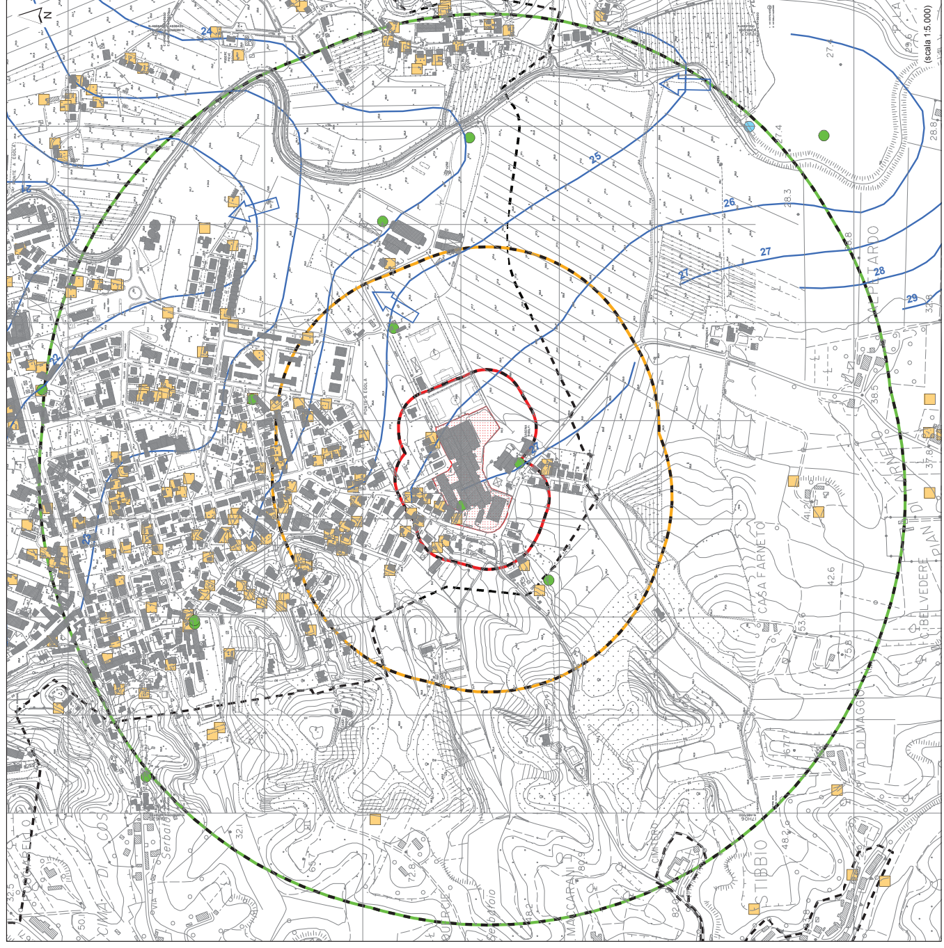
Tavola 3 Elementi ambientali nell'intorno dello stabilimento M3 srl (ex ICL A SpA) - distribuzione dei pozzi concessionari e ad uso domestico, con riportate le curve isopleze e le direzioni principali di deflusso, tratte dalla cartografia idrogeologica allegata al Piano Strutturale comunale (anno 2003)
